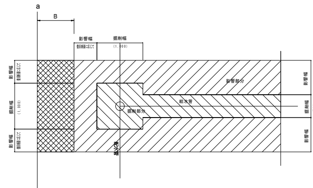
舗装復旧標準図
