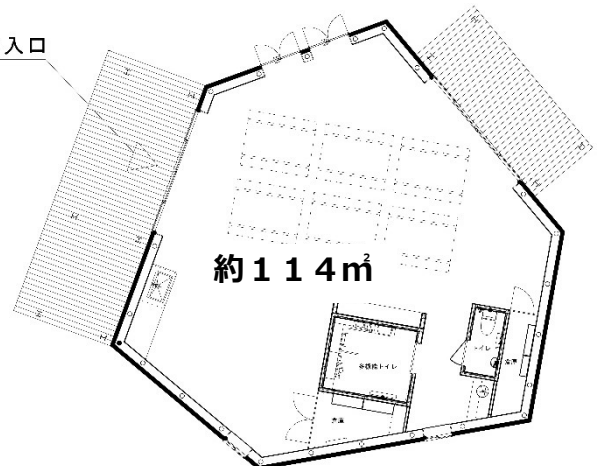
センターハウス平面図
