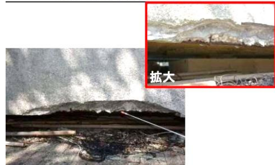
外壁 コンクリート剥落、鉄筋露出発錆
