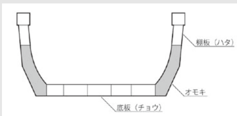
ドブネの横断面図。底板左右両側の部材がオモキです。
