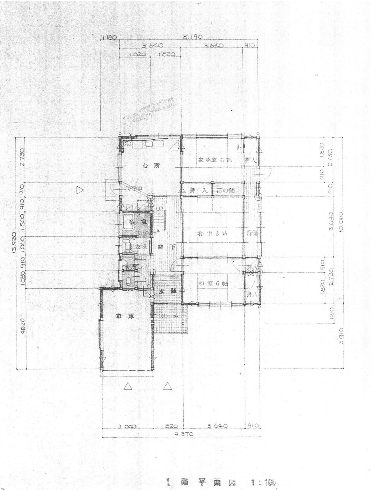
栄町医師住宅 建物平面図（中・南共通 1階）
