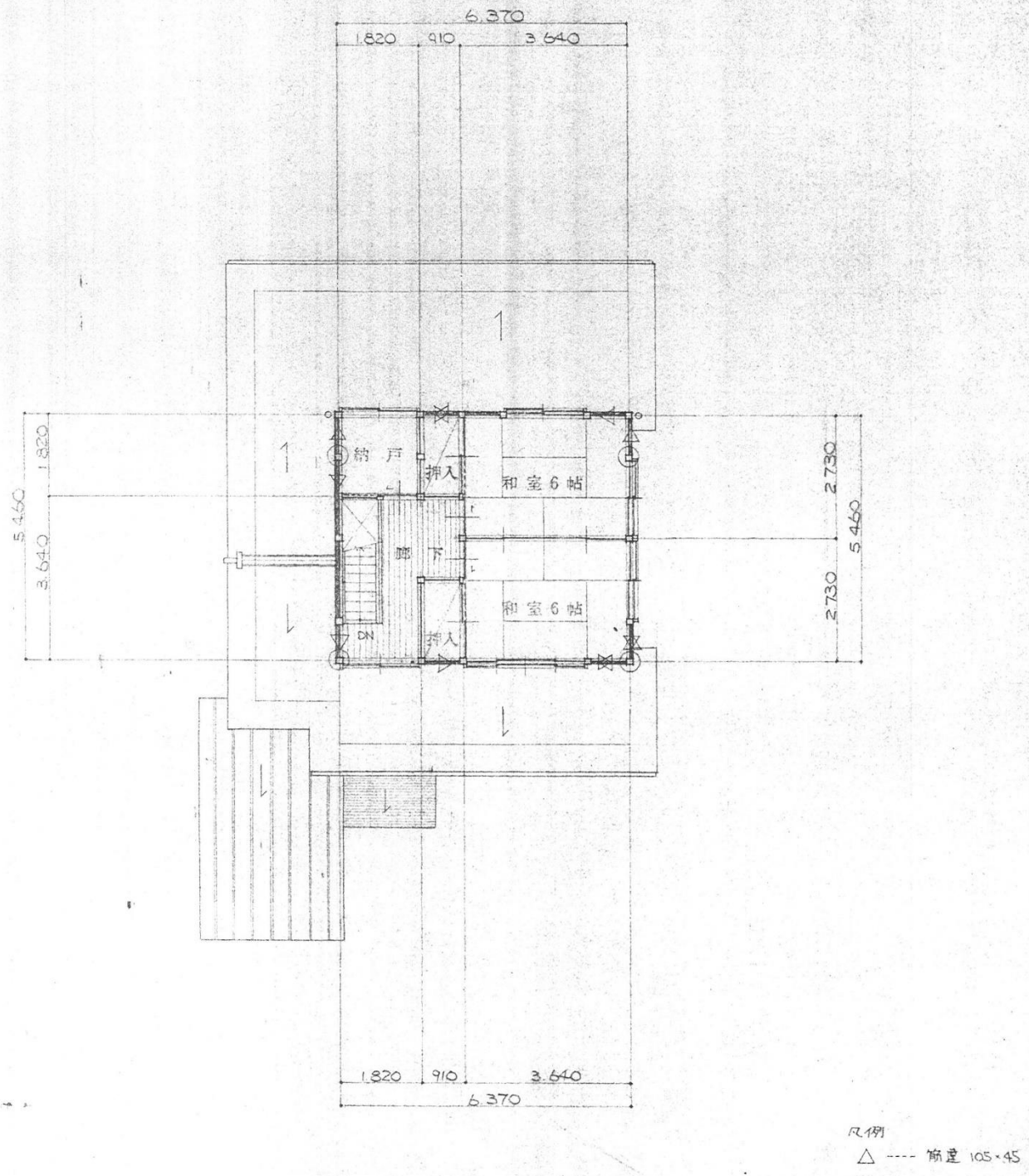
2 階 平 面 図 1:100
