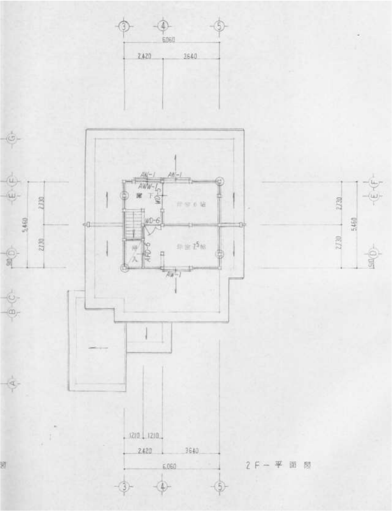
旧栄町市民病院医師住宅 建物平面図（2階）
